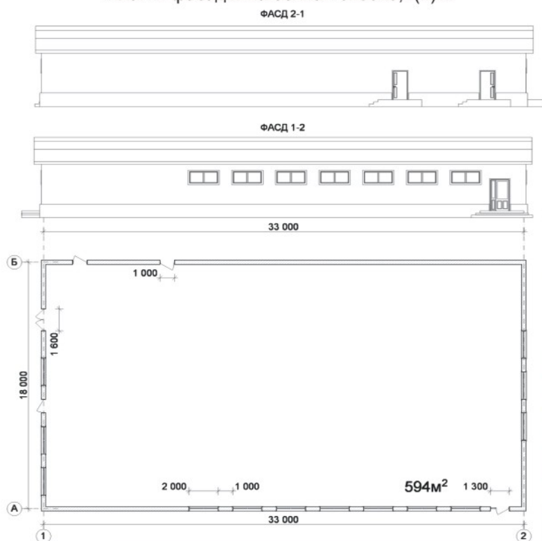
План и фасады магазина 18x33x3,4(н)м.
