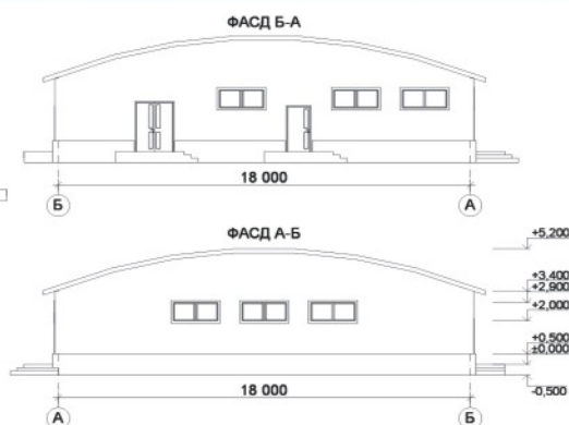
Бескаркасное здание однопролетное. Магазин 18x33x3,4(н)м.
